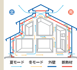
夏は上昇した熱い空気を排出。冬は家全体を暖かい空気が循環
